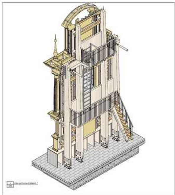
Egitura aurreratuaren eta kokapen berrian dagoeneko muntatuta dagoen erretaularen perspektiba. Atzeko bista
