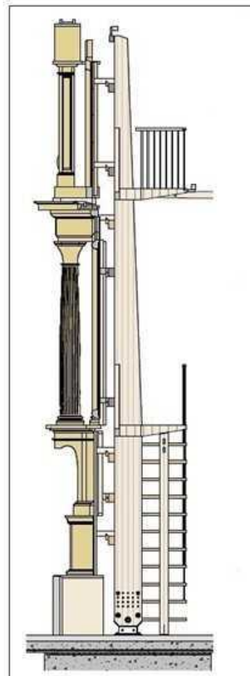
Luzetarako sekzioa. Erretaula, egurrezko oinarri batean gainean egongo da eta egurrezko egitura bati lotuko zaio
