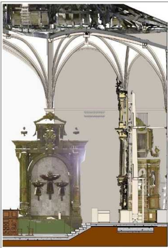
Luzetarako sekzioa. Erretaula, egurrezko oinarri batean gainean egongo da eta egurrezko egitura bati lotuko zaio
