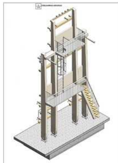
Aurreratutako egituraren perspektiba. Atzeko bista. Iturria: Landa-Ochandiano arquitectos.
